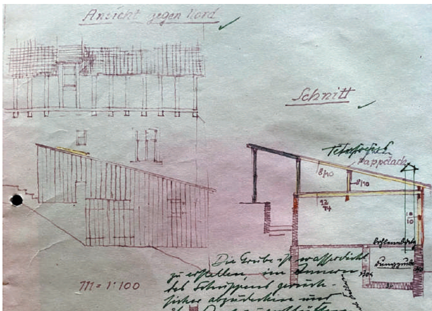
Bauplan, Ansicht von Norden, Anbau von 1939, F. Barthelmann
