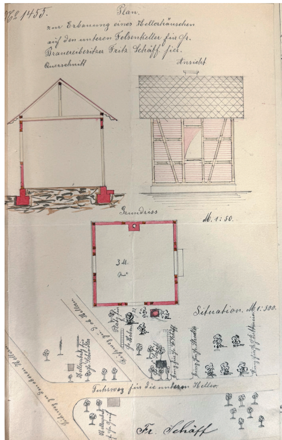
Planzeichnung zur Erbauung des unteren Schankhauses, 1896
