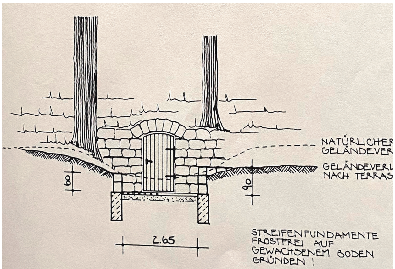
Planzeichnung zu Reparaturarbeiten am Eingang zum Felsenkeller, Behr + Gebhardt Architekten, P. Müller 1988
